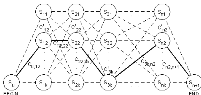
Slika 4. Pretraga govorne baze u potrazi za optimalnom sekvencom segmenata
