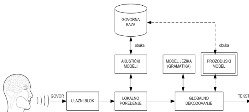
Slika 1. Blok-dijagram postupka automatskog prepoznavanja govora
