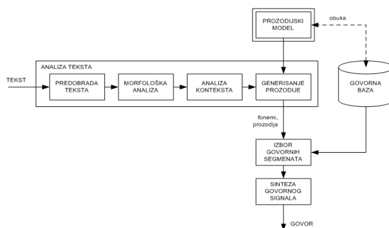
Slika 2. Blok-dijagram postupka sinteze govora na osnovu teksta
