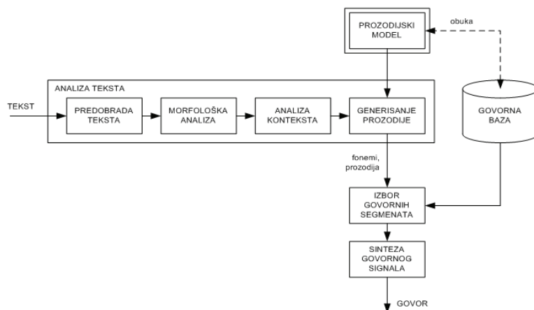
Slika 2. Blok-dijagram postupka sinteze govora na osnovu teksta
